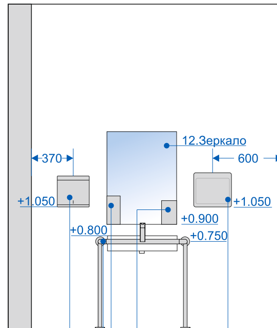
03.Мини диспенсер бумажных полотенец 01.Диспенсер для мыла 07.Сушилка для рук 11.Комплект поручней для ММГН 02.Дозатор для дезинфицирующих средств
