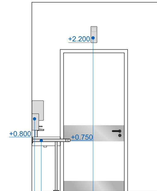
11.Комплект поручней для ММГН 08.Диспенсер для аэрозольного освежителя воздуха (центрировать относительно двери) 01.Диспенсер для мыла
