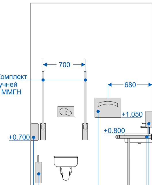
11.Комплект поручней для ММГН 06.Ерш для унитаза 04.Диспенсер туалетной бумаги 05.Диспенсер гигиенических покрытий для унитаза 02.Дозатор для дезинфицирующих средств 11.Комплект поручней для ММГН
